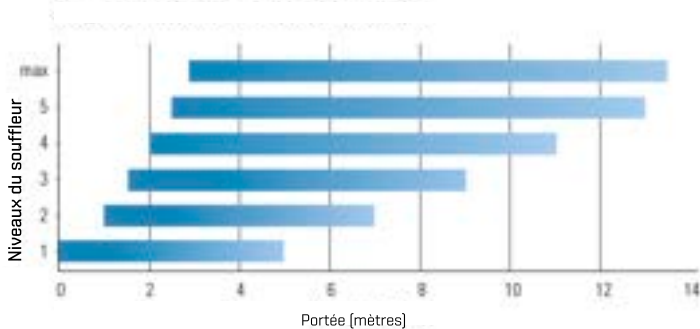
Portée en fonction de la vitesse du ventilateur
