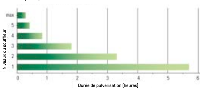
Temps de pulvérisation AS1200
